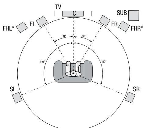
Højttalerplacering for 7.1-kanals systemer (kun AVR 1710S/AVR 171S) (I midten: med surround-bag højttalere, Nederst: med fronthøjde højttalere)
